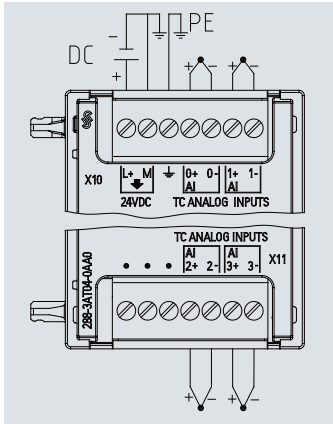
EM AT04
