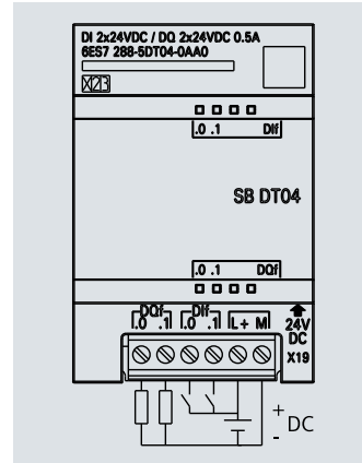
SB DT04
