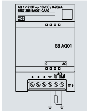
SB AQ01
